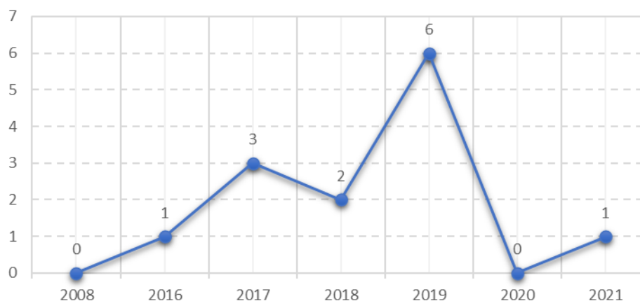
Gráfico 2 – Incidência das publicações científicas
