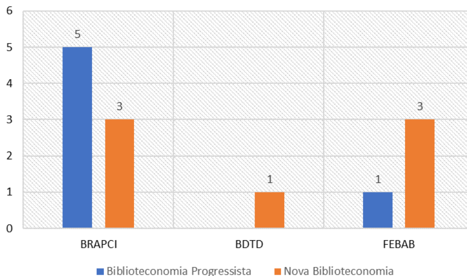
Gráfico 1 – Incidência das publicações indexadas nas bases de dados selecionadas
