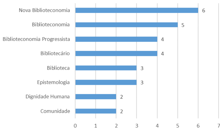
Gráfico 3 – Palavras-chave das produções indexadas
